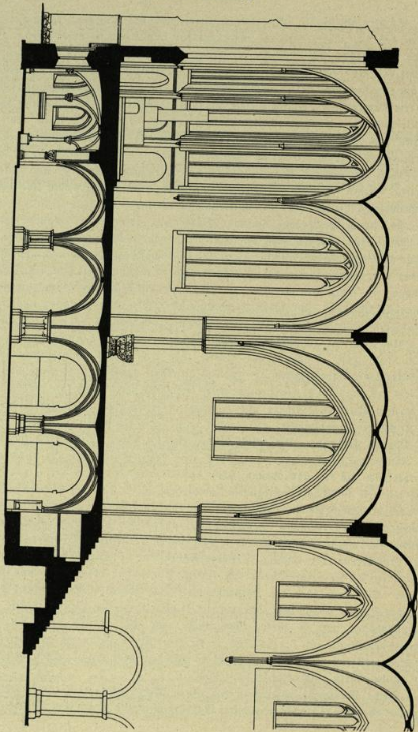
Abb. 178. Domkirche. Längsschnitt durch den Chor.
