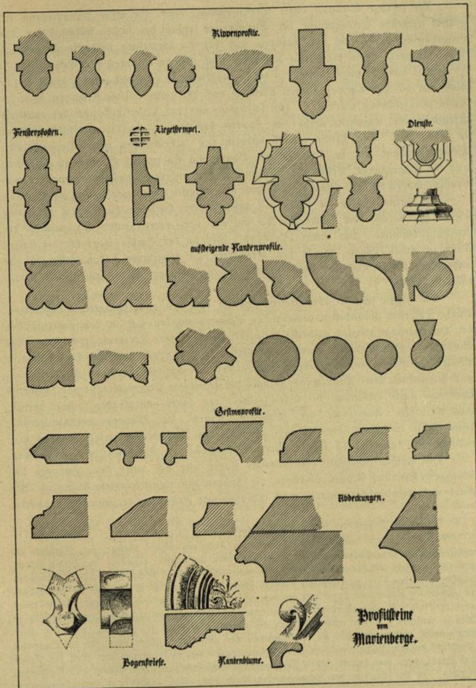
Abb. 81. Auf dem Marienberge gefundene Formsteine, die teils im Erdgeschoßraume des Kriegerdenkmals, teils im Steintorturme aufbewahrt werden (Maßstab 1:10).
