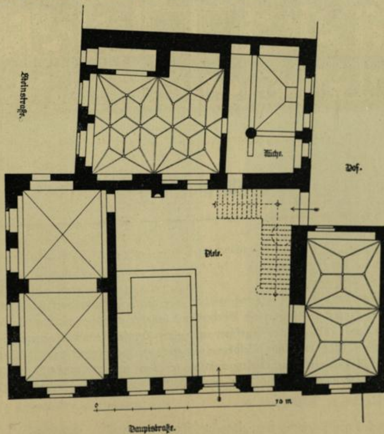
Abb. 115. Erdgeschoßgrundriß des ehemaligen Hauses Storbedt.
