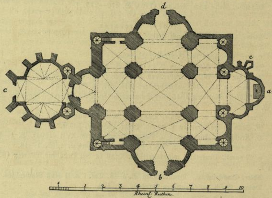
Abb. 78. Unterer Grundriß der Marienkirche (Faksimile der Heins'schen Kupferplatte).
