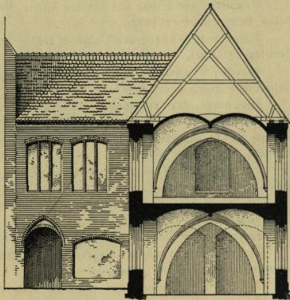
Abb. 74. Vaulikloster. Querschnitt der Bücherei mit Ansicht des Klostereingangs.
