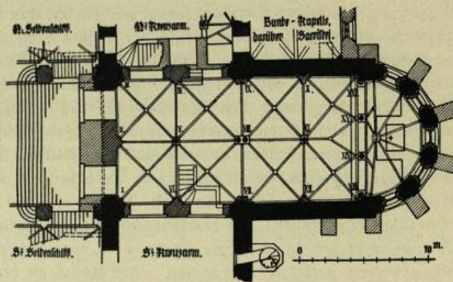
Abb. 164. Domkirche. Grundriß der Krypta.
