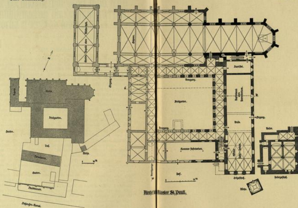
Pauliskloster. Lageplan und Erdgeschossgrundriß.
