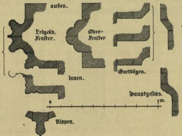
Abb. 75. Vaulikloster. Profile der Bücherei.
