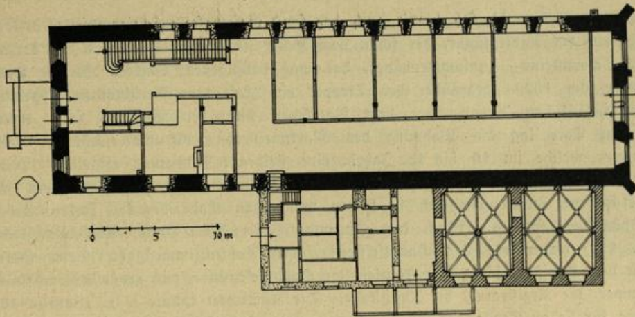
Abb. 93. Erdgeschoßgrundriß des Neustädter Rathauses (vor dem Umbau).
