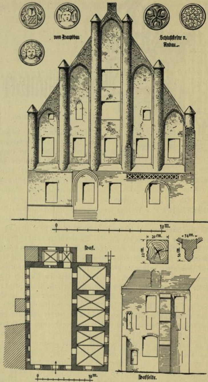
Abb. 104. Gotisches Steinhaus der Altstadt (sog. Ordnungshaus). Grundriß und Ansichten.
