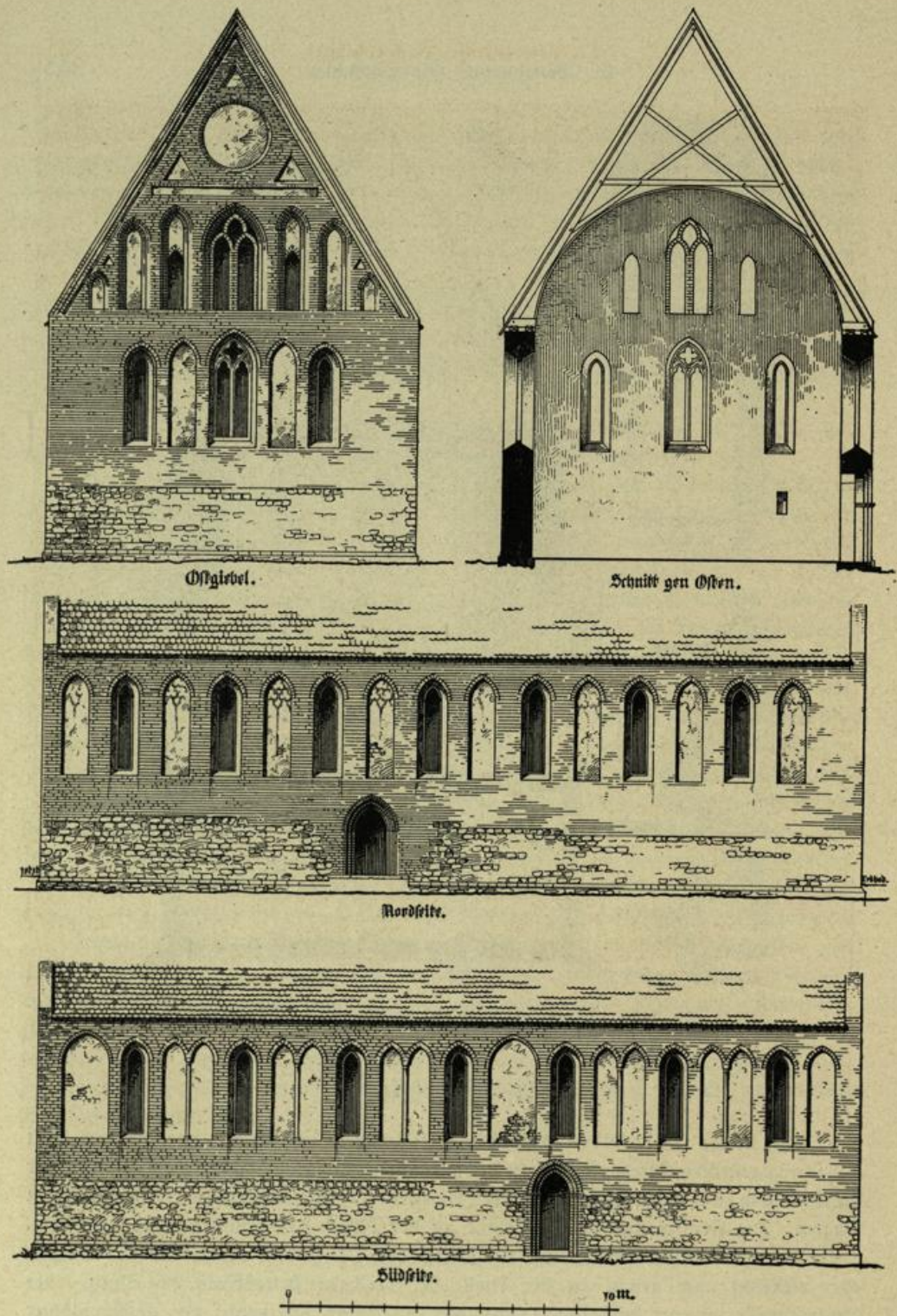
Abb. 248. Ostgiebel und Langseiten der Peterkirche nebst Schnitt mit der ursprünglichen Deckenausbildung.
