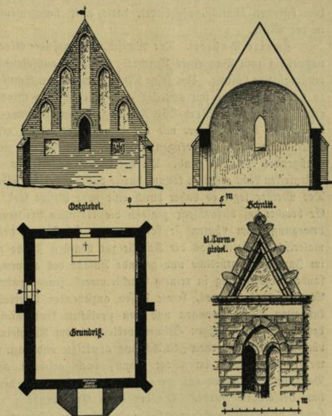
Abb. 22. Jakobskapelle. Grundriß, Schnitt, Ostgiebel und Turmfenster.
