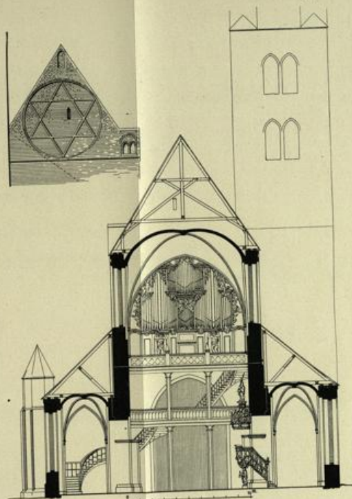
Querschnitt durch das Langhaus nebst Westgabel.
