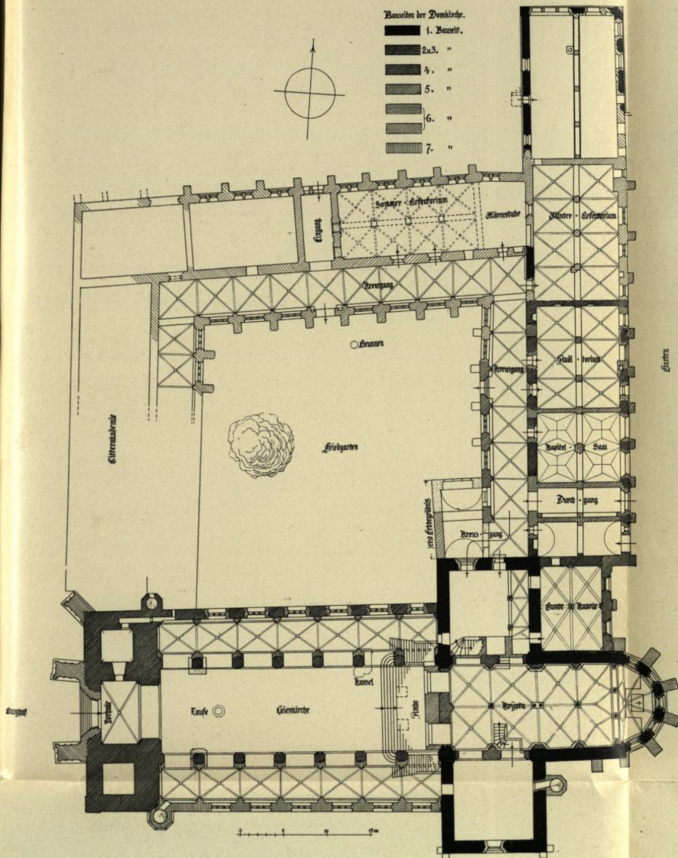
Grundriß der Domkirche und der Klausurgebäude.
