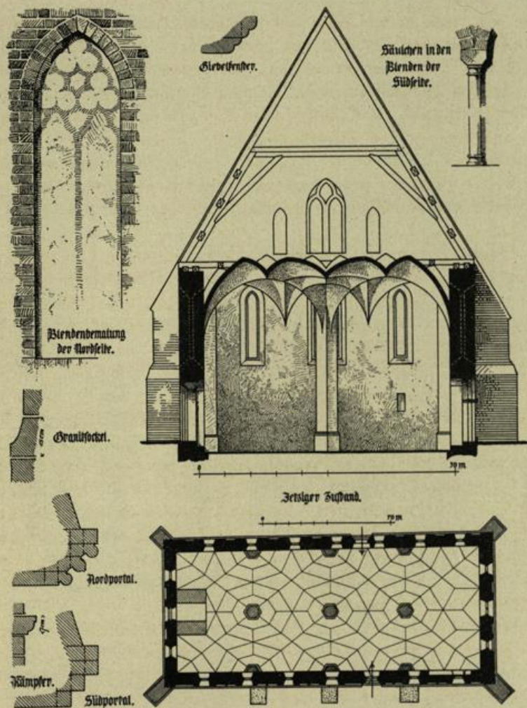
Abb. 247. Grundriß, Schnitt und Einzelheiten der Peterskirche.
