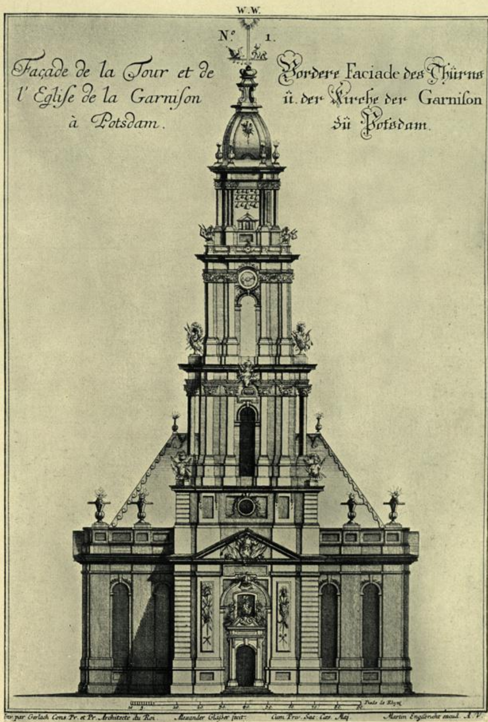
Abb. 8. Garnisonkirche, Südansicht
