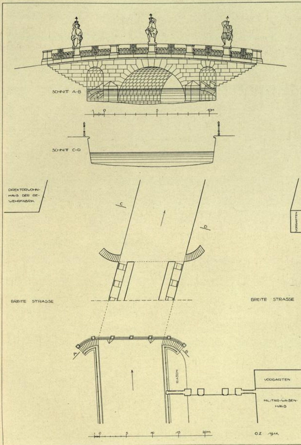
Abb. 14. Breite Brücke und Profil des Stadtkanals
