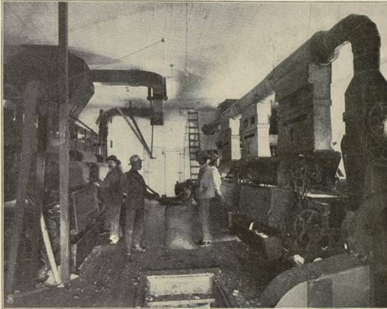
Entkörnungs- oder Ginmaschinen.
