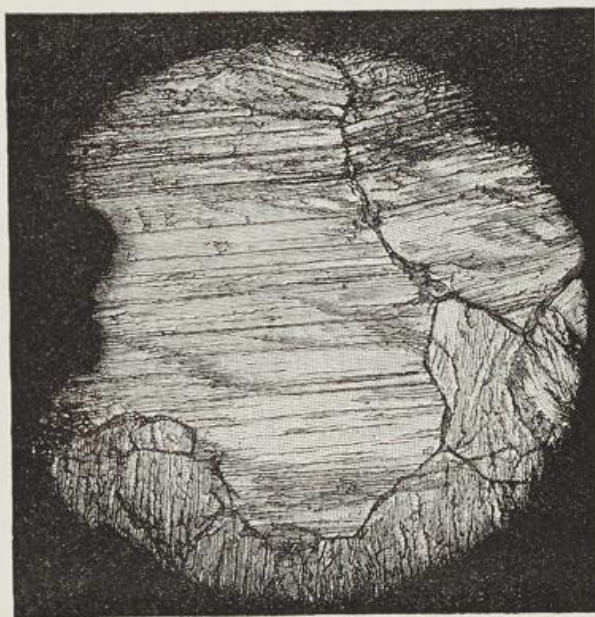
Strukturbild des Enstatits, woraus die Verschiedenheit von den Meteoritenformen zu ersehen.
